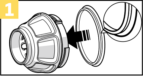
Sicherstellen, dass die breitere Seite der Verriegelungskappendichtung nach außen zeigt.
