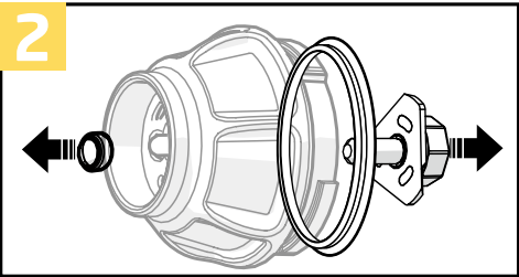
Klingenhalter, Tresterklinge und Dichtung der Verriegelungskappe entfernen. Klingenhalter sicher aufbewahren.
