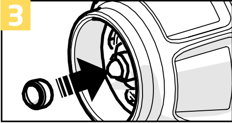
Setzen Sie die Klingenhalterung auf die aus der Verriegelungskappe herausragenden Klingenspindel. Sollte die Dichtung abhanden gekommen sein, verwenden Sie die am Boden des Motorblocks angebrachte Ersatzdichtung.
